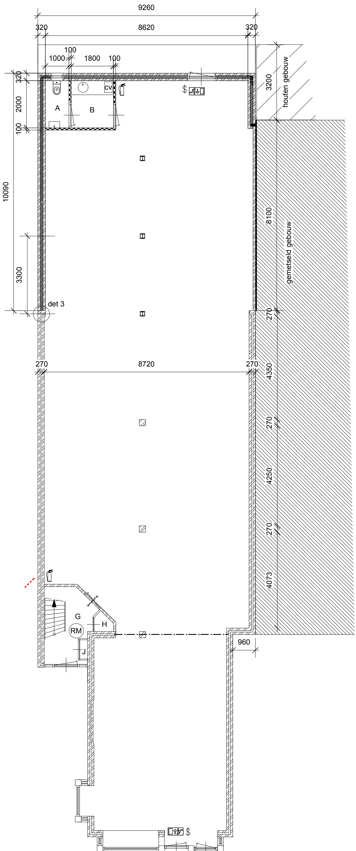
Begane Grond
